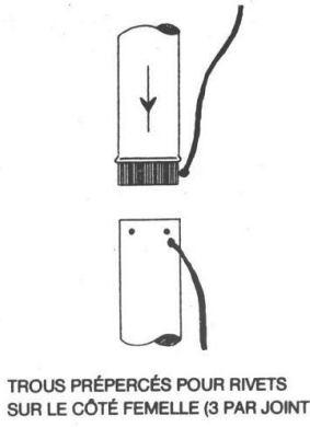
SCHÉMA 2 ASSEMBLAGE DES SECTIONS
